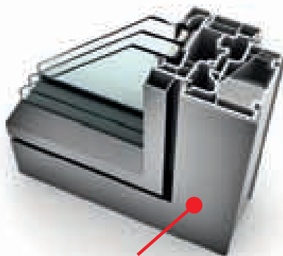
VORSATZSCHALE AUS ALUMINIUM
